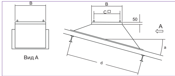
d: Расстояние между балками а: Угол наклона кровли
